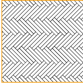
Doppel-Fischgrat
